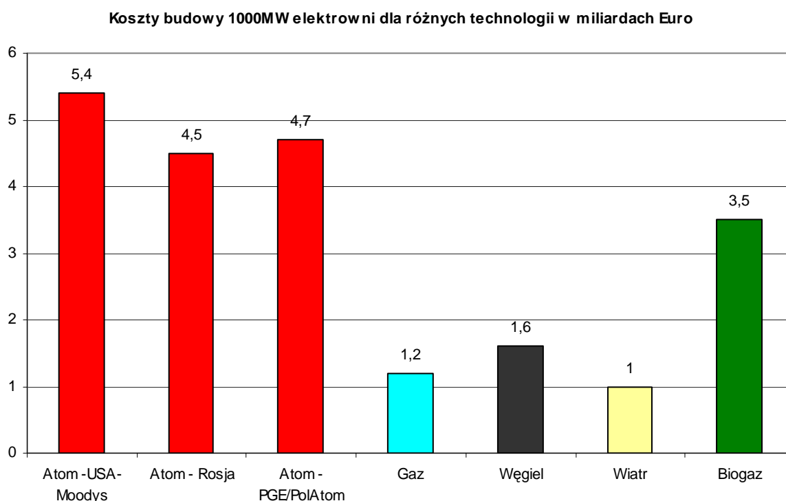
Rys. 1. Koszty inwestycyjne dla różnych technologii produkcji energii elektrycznej.
