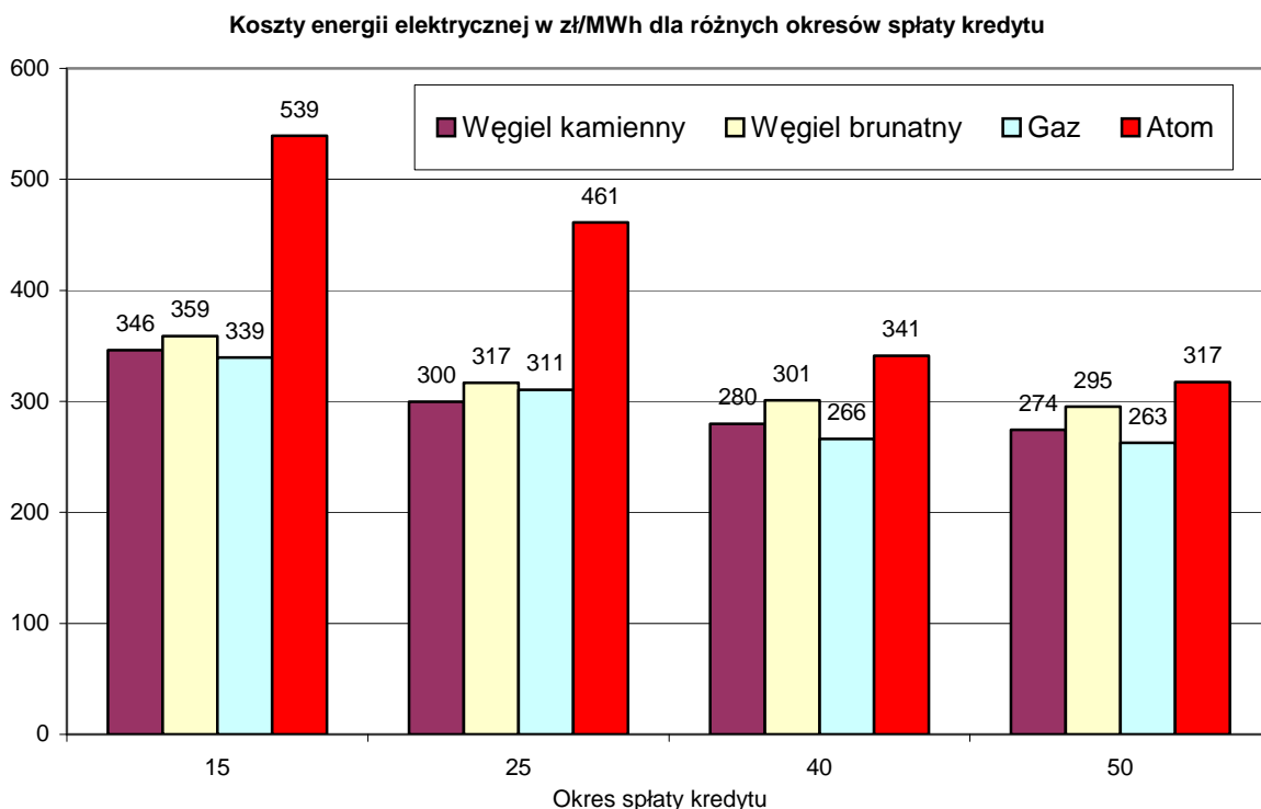
Rys. 2. Koszty produkcji energii elektrycznej dla różnych okresów spłaty kredytu.
