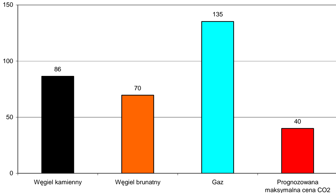
Rys. 4. Koszt emisji CO 2 dla których energii elektryczna z elektrowni atomowych jest konkurencyjna na rynku.
