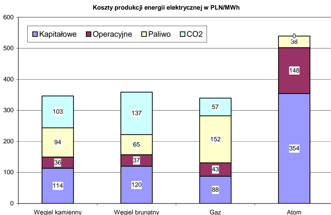
Rys. 3. Koszty produkcji energii elektrycznej z różnych technologii.
