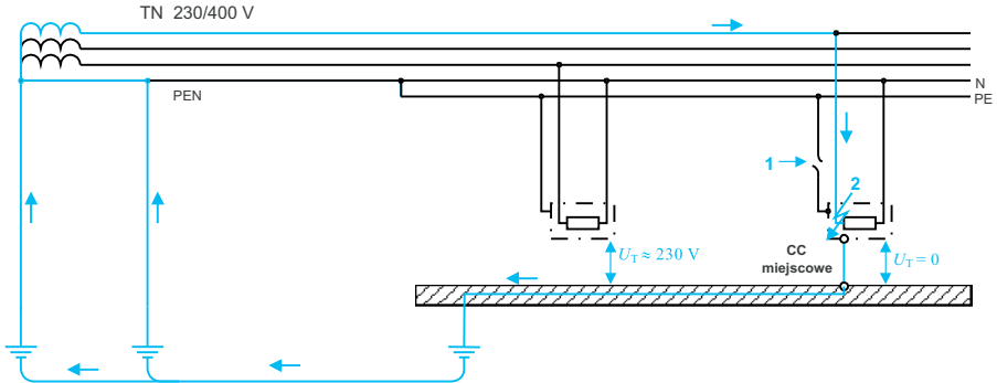
Rys. 9. Konsekwencje braku połączeń wyrównawczych głównych w sytuacji z rys. 8.
