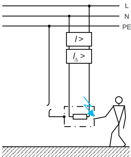
Rys. 2. Przypadek podwójnego uszkodzenia: ochrony podstawowej (przebite izolacji podstawowej) oraz ochrony dodatkowej (przerwanie przewodu ochronnego)
