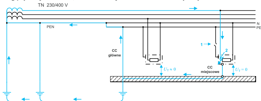
Rys. 8. Sytuacja, w której połączenia wyrównawcze zapobiegają porażeniu mimo wystąpienia podwójnego uszkodzenia
