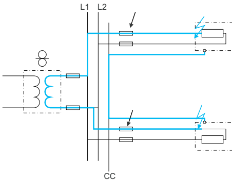
Rys. 12. Separacja ochronna dwóch lub więcej urządzeń – wymagane nieziemione połączenia wyrównawcze miejscowe Przy zwarciu dwumiejscowym, jak na rysunku, powinno zadziałać co najmniej jedno ze wskazanych zabezpieczeń nadprądowych.
