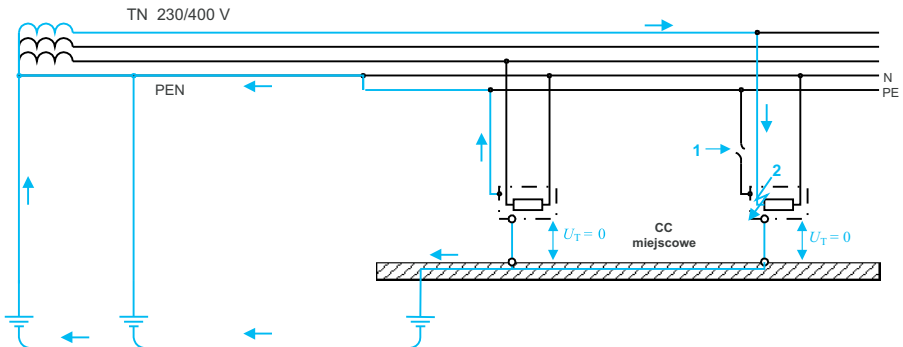
Rys. 10. Groźba przekroczenia obciążalności cieplnej przewodów połączeń wyrównawczych miejscowych przy braku połączeń wyrównawczych głównych
