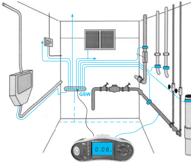
Rys. 14. Sprawdzenie ciągłości głównego połączenia wyrównawczego między głównym rurociągiem wody a główną szyną wyrównawczą w pomieszczeniu przyłączowym budynku
