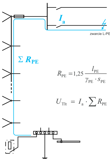
Rys. 11. Sposób obliczania największego występującego długotrwale napięcia dotykowego w wielopiętrowym budynku
