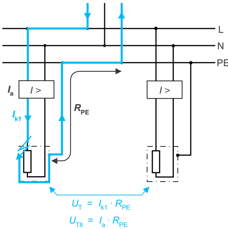
Rys. 1. Ekwipotentjalizujący efekt połączeń ochronnych PE w przypadku uszkodzenia izolacji podstawowej w jednym z odbiorników
