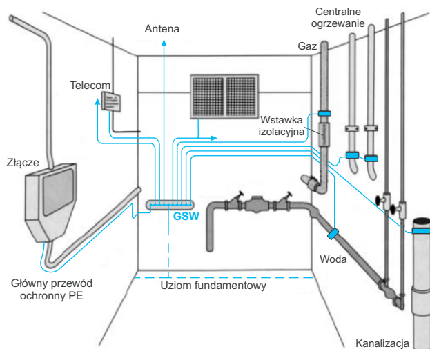
Rys. 4. Główne połączenia wyrównawcze w pomieszczeniu przyłączowym budynku
