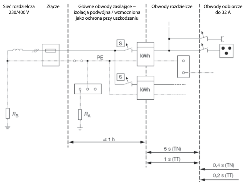
Rys. 47. Wymagany czas SWZ w instalacji odbiorczej o układzie TN i TT
