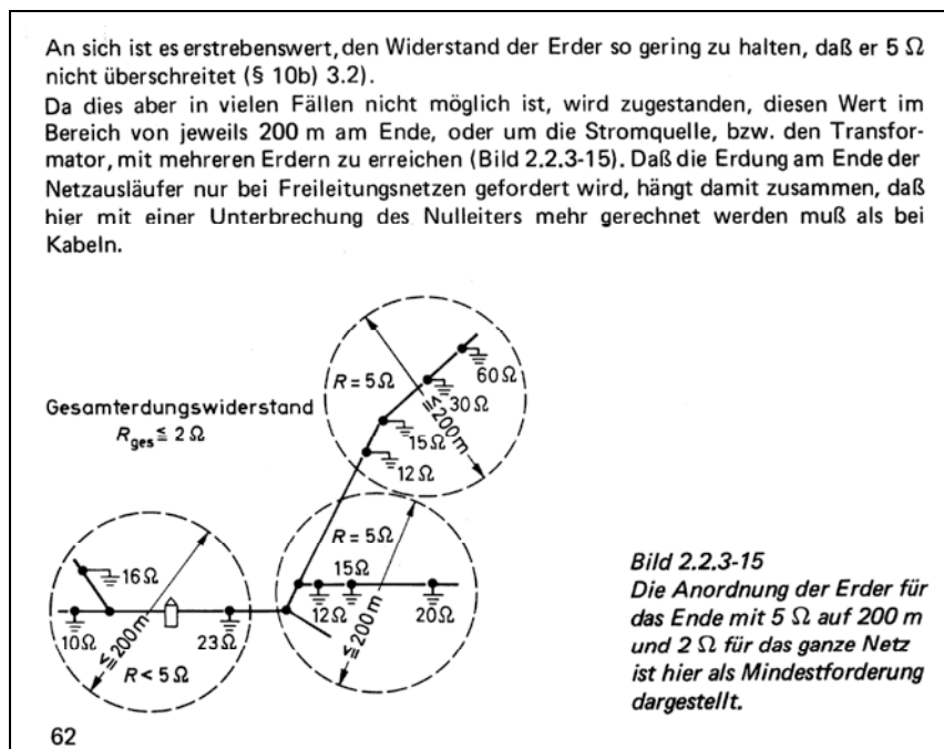
Rys. 36. Wymagania przepisów niemieckich VDE 0100/11.58 z roku 1958 odnośnie do rozmieszczenia i rezystancji uziemień ochronno-funkcjonalnych napowietrznej sieci przystosowanej do zerowania [6]
