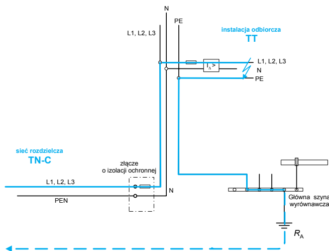
Rys. 52. Wyspa TT w sieci TN – obwód prądu zwarcia doziemnego L-PE w instalacji odbiorczej
