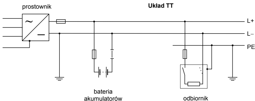
Rys. 25. Instalacja stałoprądowa o układzie TT
