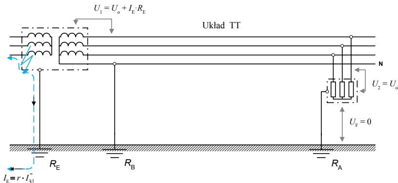
Rys. 30. Oddzielne uziemienie ochronne urządzeń SN stacji i uziemienie funkcjonalne sieci nn o układzie TT – narażenia napięciowe izolacji urządzeń nn w stacji i u odbiorcy przy zwarcu doziemnym w urządzeniu SN w stacji
