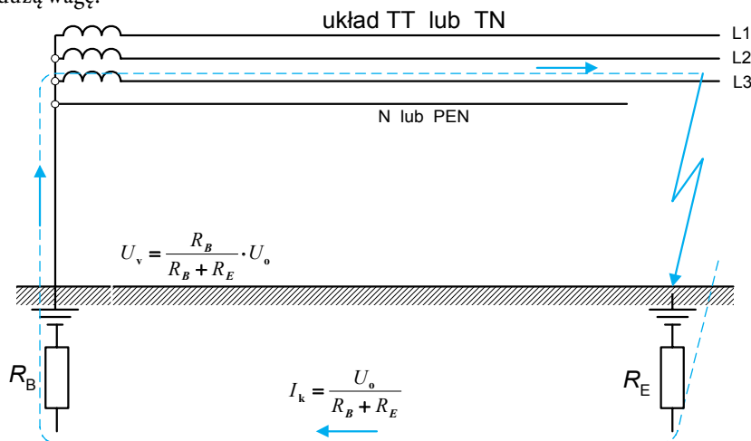
Rys. 26. Zwarcie doziemne przewodu skrajnego w sieci z uziemieniem funkcjonalnym wywołujące przesunięcie potencjału punktu neutralnego układu względem ziemi ( U_v )
