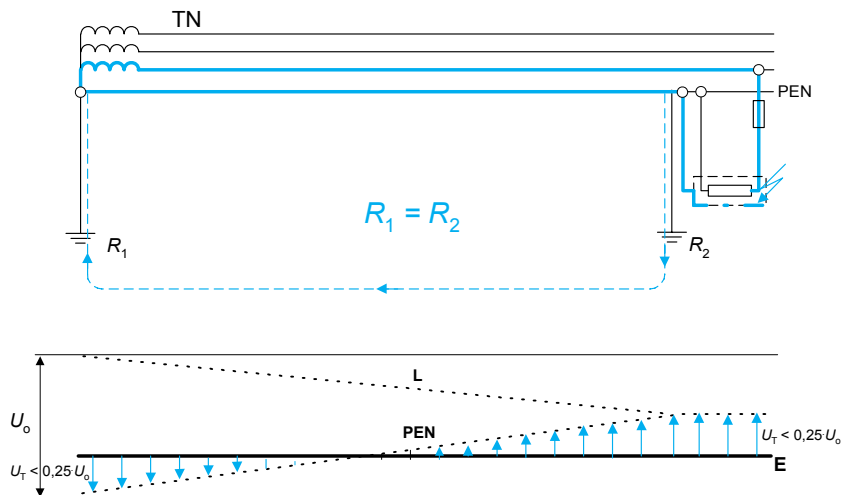
Rys. 38. Rozkład napięcia przewodu PEN względem ziemi (E) wzdłuż linii o jednakowej rezystancji uziemień ochronno-funkcyjnych na początku i na końcu
