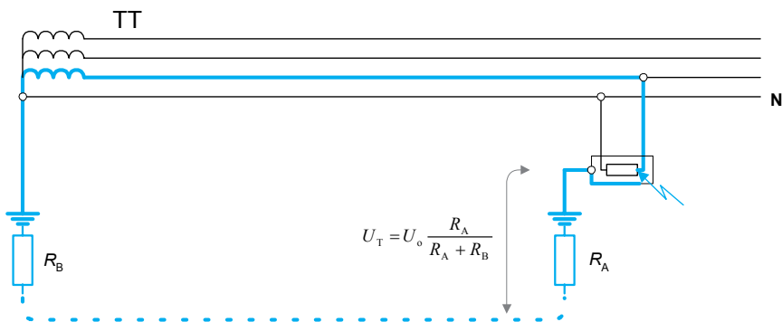
Rys. 23. Napięcie dotykowe spodziewane U_T przy uszkodzeniu izolacji podstawowej w układzie TT
