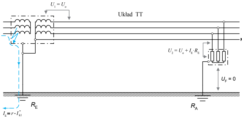
Rys. 29. Wspólne uziemienie ochronne urządzeń SN stacji i uziemienie funkcjonalne sieci nn o układzie TT – narażenia napięciowe izolacji urządzeń nn w stacji i u odbiorcy przy zwarcu doziemnym w urządzeniu SN w stacji
