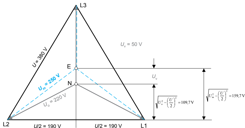
Rys. 27. Dawniejsza relacja między różnymi napięciami przy zwarciu z ziemią, jak na rys. 26, w sieci 220/380 V o bezpośrednio uziemionym punkcie neutralnym
