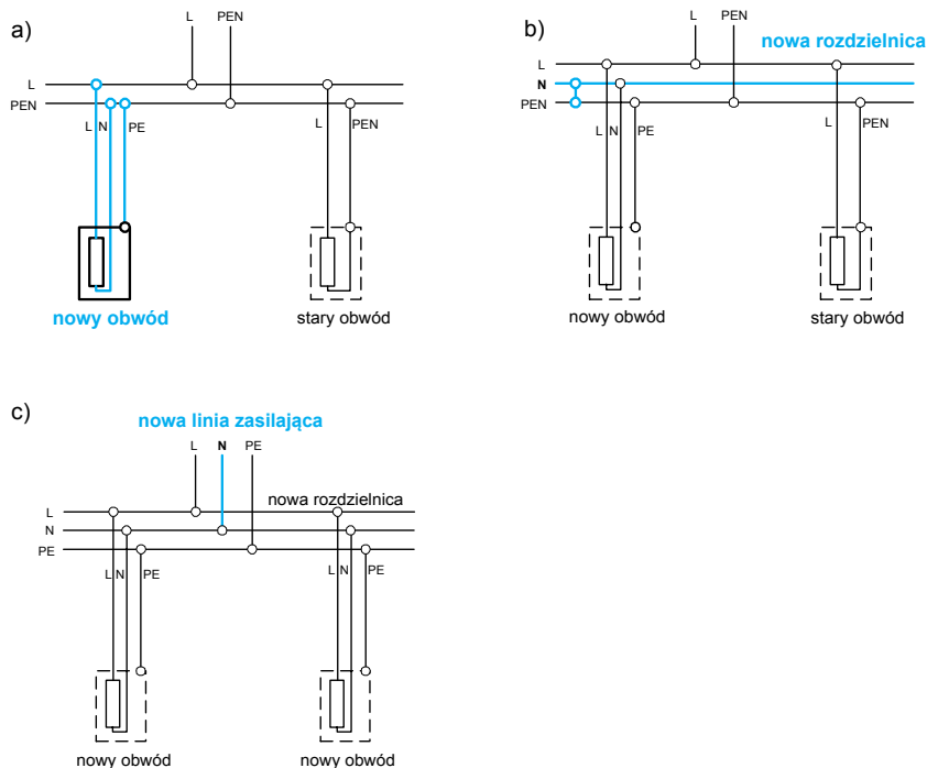
Rys. 50. Stopniowe przechodzenie z układu TN-C do układu TN-S
