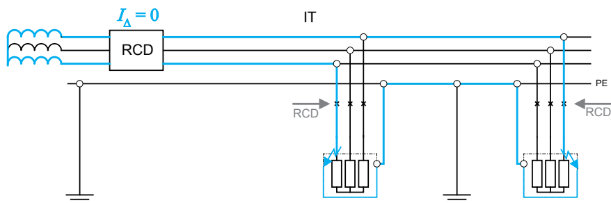
Rys. 19. Przykładowa pętla zwarcia dwumiejscowego w układzie IT
