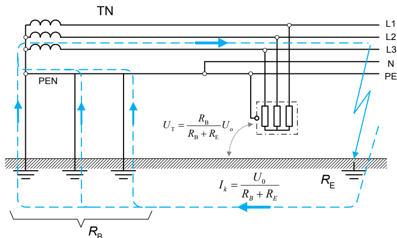
Rys. 40. Skutki zwarcia przewodu skrajnego z ziemią (L-E) w układzie TN
