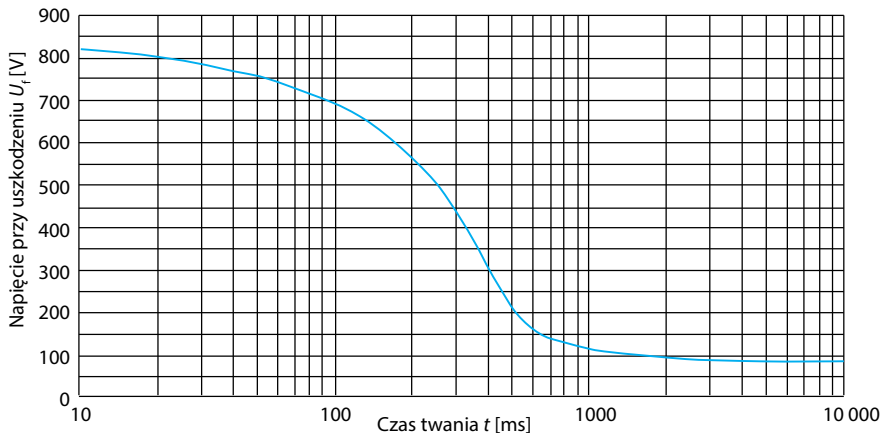
Rys. 45. Największe dopuszczalne napięcie w miejscu uszkodzenia U_f w urządzeniach niskiego napięcia w zależności od czasu trwania zwarcia doziemnego t_f w poprzedzających urządzeniach średniego napięcia [27]
