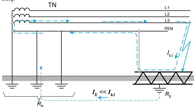
Rys. 43. Sposób eliminacji zagrożenia w przypadku, kiedy rezystancja przejścia R_E jest bardzo mała
