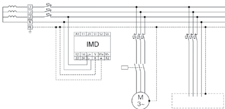
Rys. 14. Jeden ze sposobów przyłączenia urządzenia IMD do monitorowania stanu izolacji doziemnej w sieci IT
