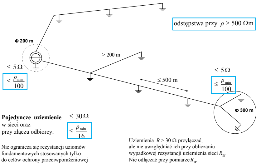
Rys. 37. Wymagania normy N SEP-E-001 [33] odnośnie do rozmieszczenia i rezystancji uziemień ochronno-funkcyjnych napowietrznej sieci TN
