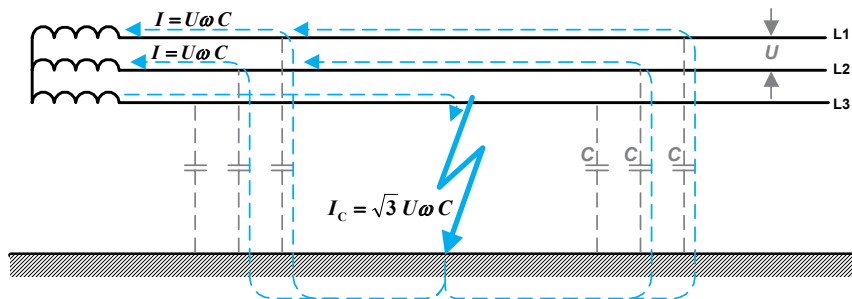
Rys. 3. Rozpływ prądu ziemnozwarciowego w sieci o izolowanym punkcie neutralnym
