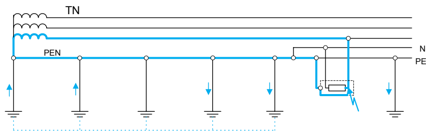
Rys. 31. Pętla zwarcia L-PE w układzie TN w całości złożona z przewodów
