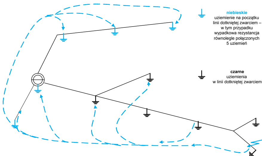
Rys. 39. Rozpływ prądu ziemnowrotnego przy zwarciu L-PEN u końca jednej z wielu linii sieci TN
