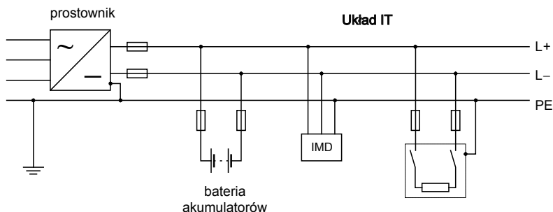
Rys. 11. Przykład instalacji prądu stałego o układzie IT, uziemienie zbiorowe części przewodzących dostępnych
