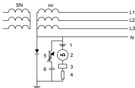
Rys. 13. Główne elementy składowe urządzenia IMD monitorującego stan izolacji doziemnej 1 – źródło napięcia stałego, 2 – miernik rezystancji izolacji doziemnej instalacji, 3 – przekaźnik uruchamiający sygnalizację doziemienia bądź wyłączenie instalacji, 4 – rezystor ograniczający prąd rażeniowy przy dotyku bezpośrednim; 5 – dławik nastawny, 6 – kondensator blokujący składową stałą
