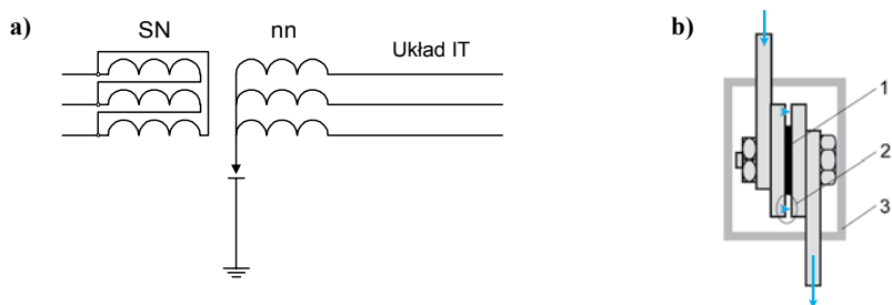
Rys. 12. Bezpiecznik iskiernikowy stosowany do ochrony przeciwprzepięciowej układu IT zasilanego przez transformator z sieci wysokiego napięcia: a) umiejscowienie; b) zasada budowy 1 – warstwa izolacyjna niszczona przez przepięcie o dużej energii, 2 – strefa zapłonu przy przepięciu o małej energii, 3 – obudowa izolacyjna
