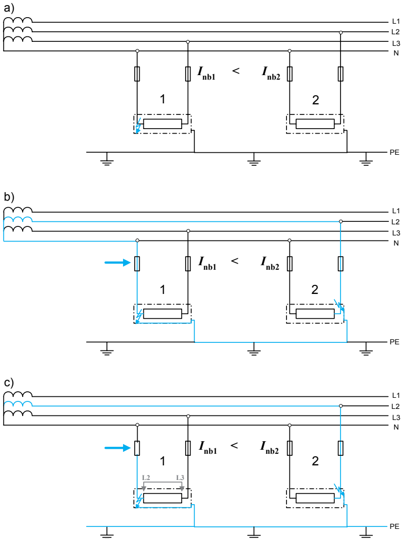
Rys. 20. Następstwa niepełnobiegunowego wyłączenia dwumiejscowego zwarcia w układzie IT z rozproszonym przewodem neutralnym:
