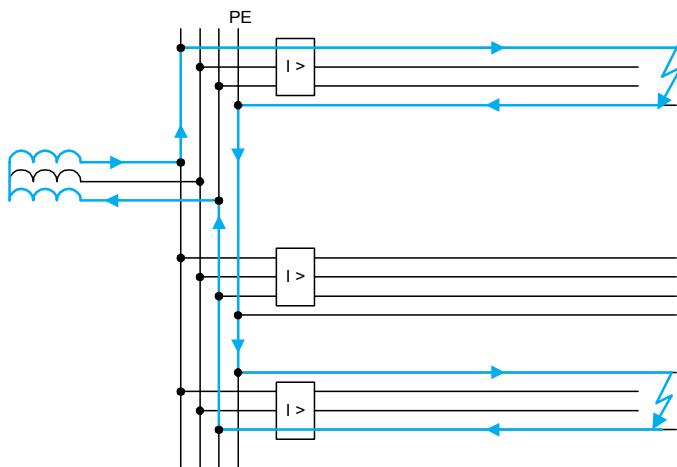
Rys. 17. Przykładowa pętla zwarcia dwumiejscowego w układzie IT
