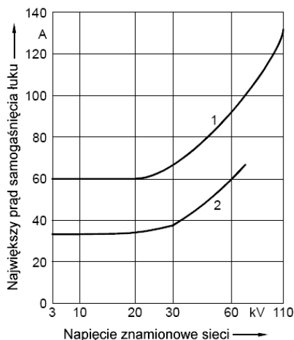
Rys. 5. Graniczny prąd samogaśnięcia łuku w zależności od napięcia znamionowego sieci napowietrznej: 1 – skompensowanej, 2 – o izolowanym punkcie neutralnym
