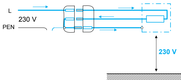
Rys. 34. Skutki przerwania przewodu ochronno-neutralnego PEN w instalacji o układzie TN-C
