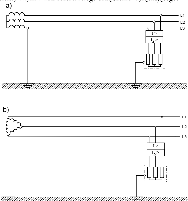
Rys. 24. Przykłady nietypowych układów TT: a) niedostępny punkt neutralny układu zasilania; b) brak naturalnego punktu neutralnego układu zasilania (ang. corner-earthed system)
