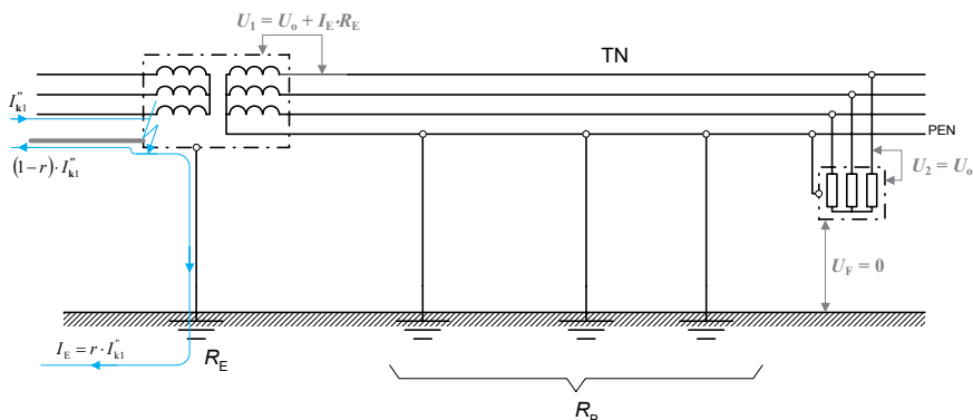
Rys. 46. Skutki zwarcia doziemnego po stronie SN stacji SN/nn o oddzielnych uziemieniach dla urządzeń średniego napięcia i urządzeń niskiego napięcia
