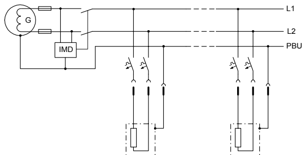
Rys. 21. Instalacja o układzie IT zasilana z przewodowego zespołu spaliniowo-elektrycznego z urządzeniem IMD pobudzającym wyłączenie po pierwszym uszkodzeniu izolacji
