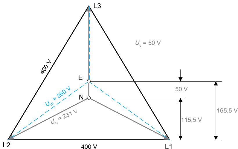
Rys. 28. Aktualna relacja między różnymi napięciami przy zwarciu doziemnym, jak na rys. 26, w sieci 230/400 V o bezpośrednio uziemionym punkcie neutralnym
