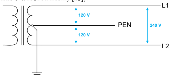
Rys. 32. Jednofazowy trzyprzewodowy układ TN (multi-grounded neutral system) 120/240 V, 60 Hz w USA
