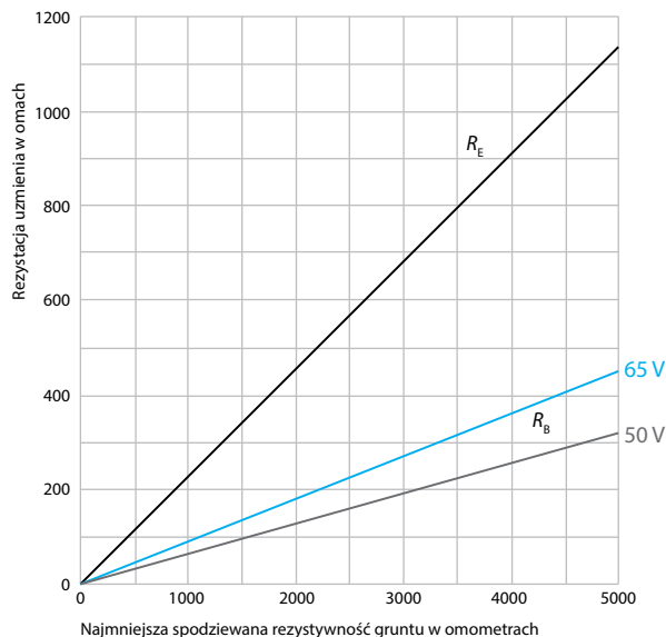
Rys. 41. Rezystancja uziemienia R_E zerwanego gołego przewodu linii napowietrznej oraz wymagana rezystancja uziemienia ochronno-funkcjonalnego R_B sieci 230/400 V w zależności od najmniejszej rezystywności gruntu na trasie linii. Wartości R_B podano dla największego dopuszczalnego długotrwale napięcia dotykowego 65 V (Austria) i 50 V (Polska). Zakres zmienności rezystywności gruntu 0 \div 5000 \Omega\text{m}
