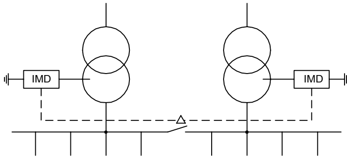
Rys. 16. Przykład blokady zapobiegającej jednoczesnej pracy dwóch urządzeń IMD w jednej galwanicznie połączonej sieci o układzie IT
