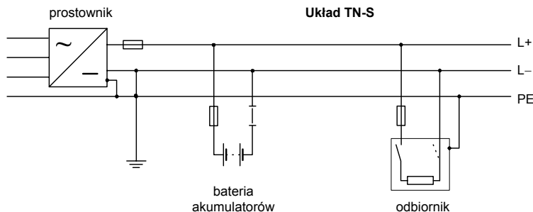
Rys. 33. Instalacja prądu stałego o układzie TN-S
