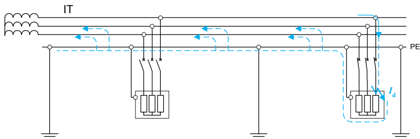
Rys. 10. Pierwsze zwarcie doziemne L-PE w układzie IT
