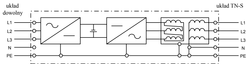
Rys. 48. Bezprzerwowo zasilacz statyczny UPS z transformatorem oddzielającym. Układ instalacji pierwotnej zasilającej UPS – dowolny, układ instalacji wtórnej – TN-S
