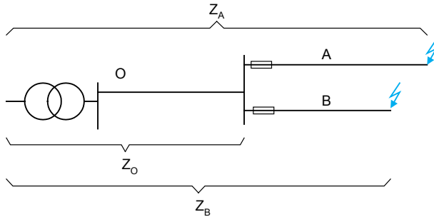
Rys. 18. Zwarcie dwumiejscowe na końcach obwodów A i B poprzedzonych wspólnym torem zasilania O
