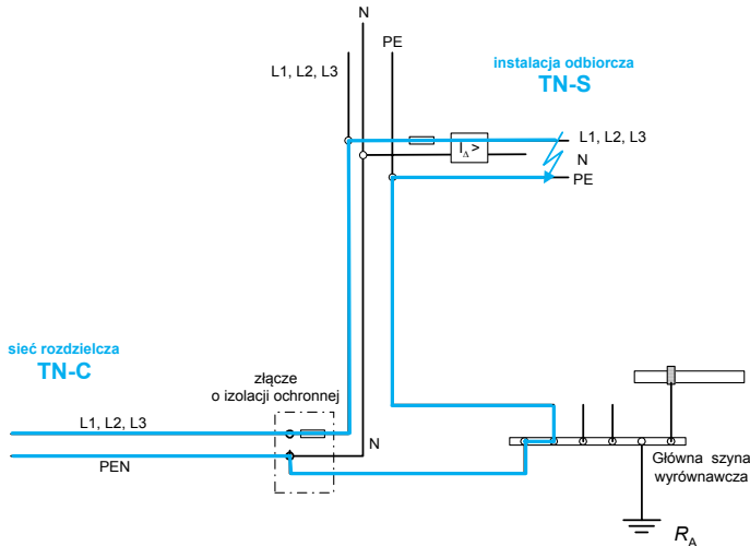
Rys. 53. Likwidacja wyspy TT w sieci TN przez połączenie przewodu ochronnego (PE, PEN) zasilającej sieci TN z główną szyną wyrównawczą instalacji odbiorczej obiektu
