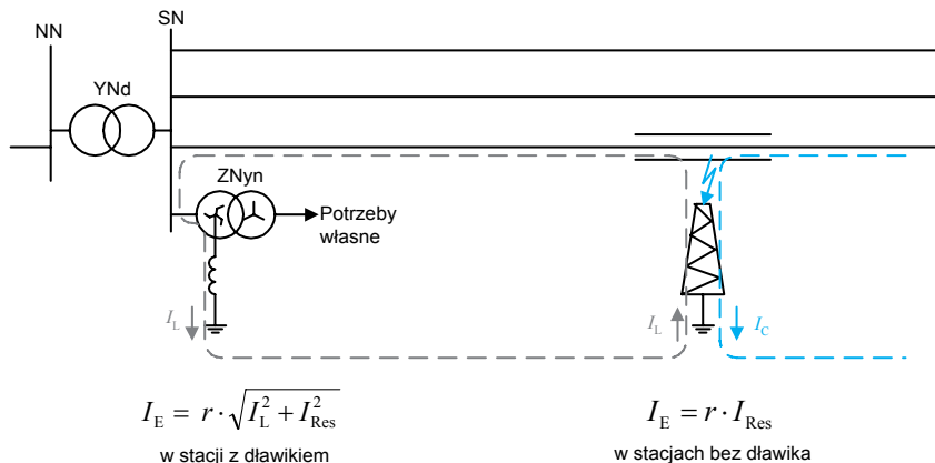
Rys. 4. Zwarcie doziemne w sieci skompensowanej: dwie składowe prądu zwarciovego w miejscu zwarcia oraz wartości prądu uziomowego I_E stanowiące podstawę wymiarowania uziemień ( r – współczynnik redukcyjny)
