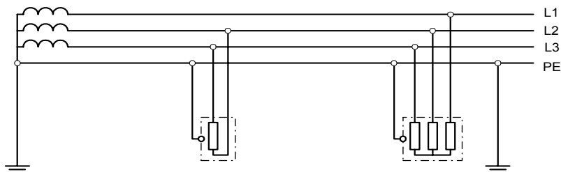
Rys. 35. Trójfazowa czteroprzewodowa instalacja o układzie TN-S
