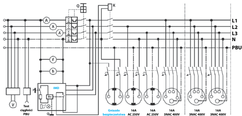
Rys. 22. Instalacja o układzie IU zasilana z przewoźnego zespołu spalinowo-elektrycznego wozu strażackiego
