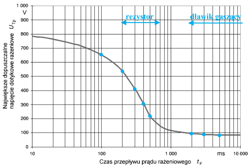
Rys. 8. Wpływ sposobu uziemienia punktu neutralnego sieci SN na wartość największego dopuszczalnego napięcia dotykowego rażeniowego przy projektowaniu uziemień
