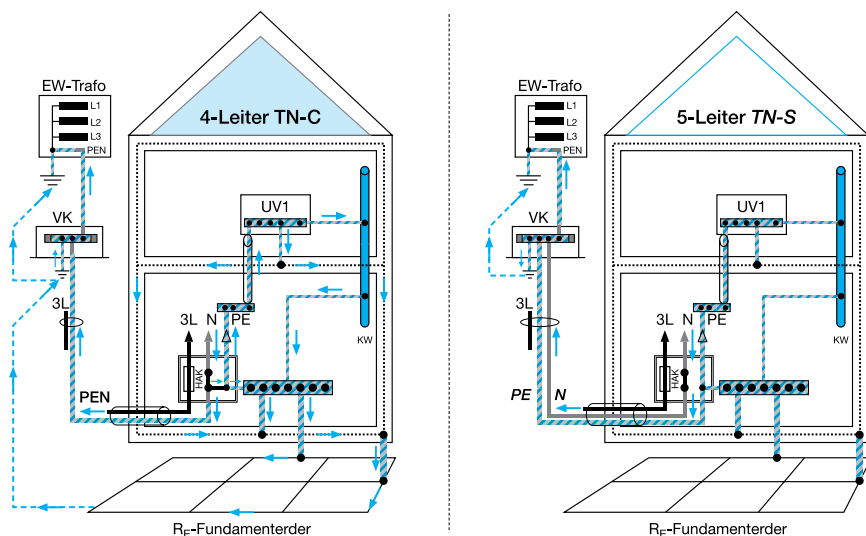
Rys. 51. Porównanie instalacji o przyłączy 4-przewodowym (a) z instalacją o przyłączy 5-przewodowym (b) [8]
