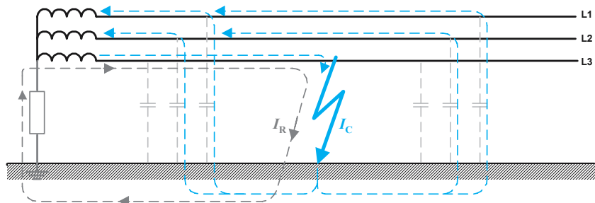
Rys. 6. Zwarcie doziemne w sieci o punkcie neutralnym uziemionym przez rezystor: dwie składowe prądu zwarciovego w miejscu zwarcia
