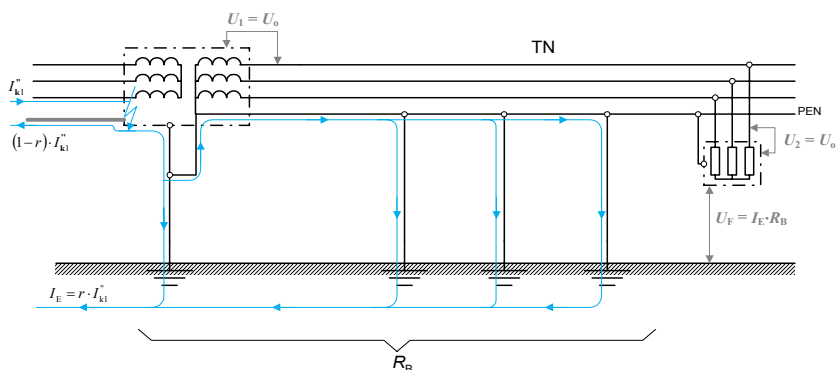
Rys. 44. Skutki zwarcia doziemnego po stronie SN stacji SN/nn o wspólnym uziemieniu dla urządzeń średniego napięcia i urządzeń niskiego napięcia
