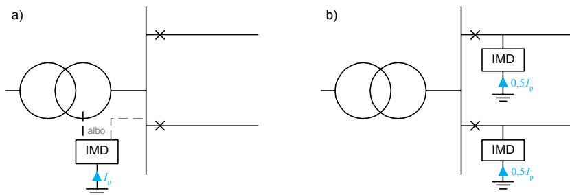
Rys. 15. Instalowanie IMD w układzie IT o dwóch liniach rozdzielczych: a) prawidłowe; b) błędne
