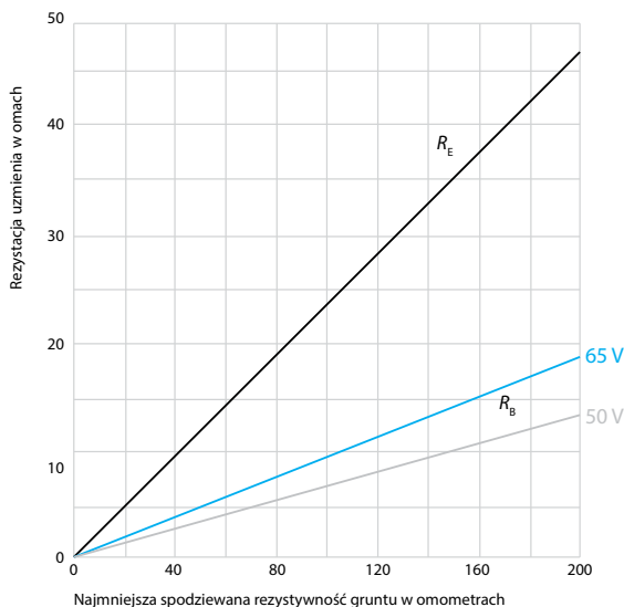
Rys. 42. Rezystancja uziemienia R_E zerwanego gołego przewodu linii napowietrznej oraz wymagana rezystancja uziemienia ochronno-funkcjonalnego R_B sieci 230/400 V w zależności od najmniejszej rezystywności gruntu na trasie linii. Wartości R_B podano dla największego dopuszczalnego długotrwale napięcia dotykowego 65 V (Austria) i 50 V (Polska). Zakres zmienności rezystywności gruntu 0 \div 200 \Omega m
