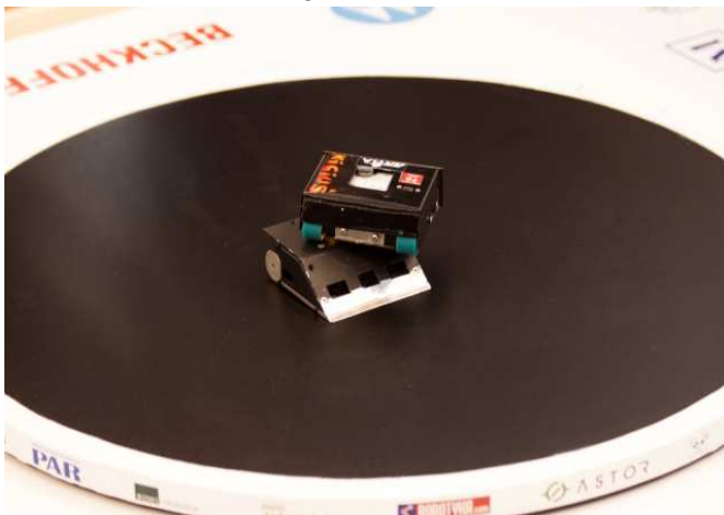
Fot. 1. Roboty walczące w kategorii minisumo.
