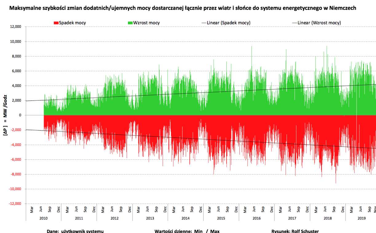
Rys. 4. Maksymalne szybkości zmian prędkości wiatru w ciągu roku w Niemczech. W każdym kwartale wykres jest efektem pomiarów ponad 40 000 chwilowych prędkości wiatru. Moc jest proporcjonalna do 3 potęgi prędkości wiatru. Zrównoważenie tych zmian przez system elektroenergetyczny jest bardzo trudne i kosztowne. Dane przedstawione przez Rolfa Schustera z NGO Vernunftkraft, cytowane za zezwoleniem
