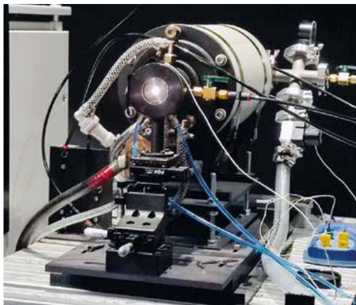
Praktyczna realizacja ciała czarnego w Laboratorium CARLO firmy GL Optic
