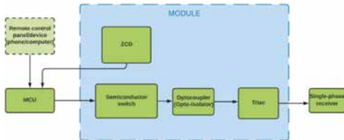
Rys. 2. Schemat blokowy modułu sterowania i jego otoczenia
